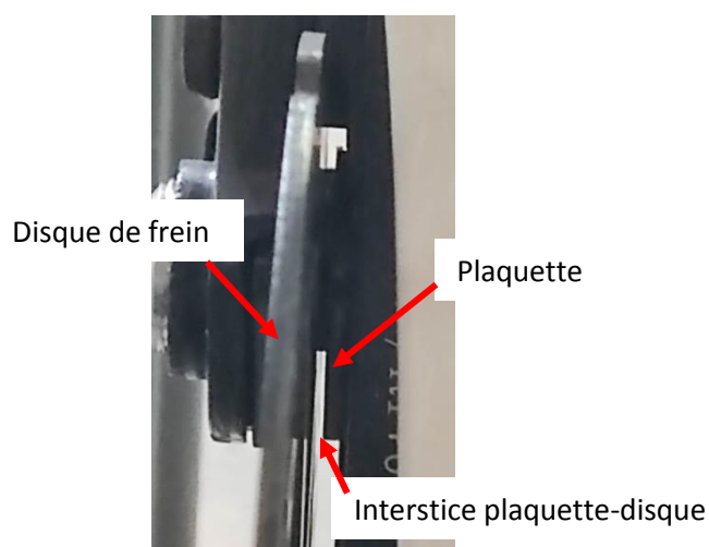
Photo 4.13 : vue avant droite du même frein
